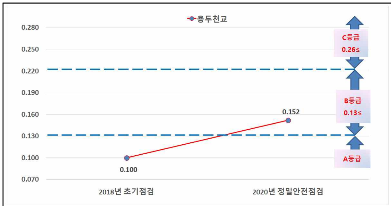
[그림 5.4.1] 용두천교 상태평가 결과 비교 그래프
